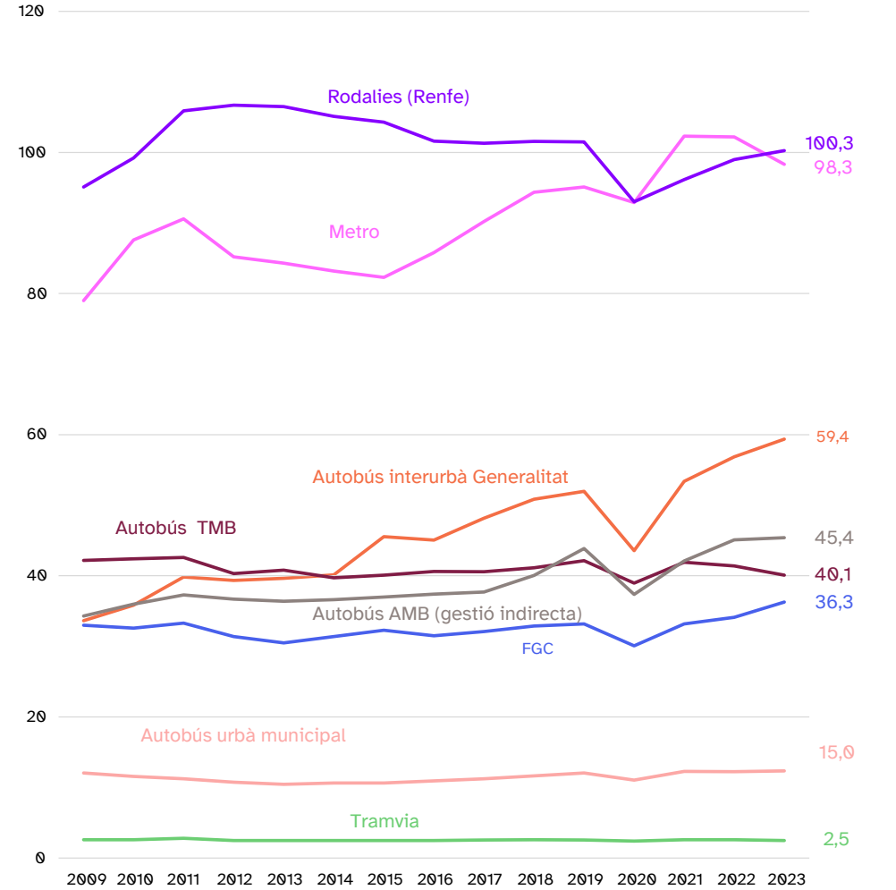
Vehicles-km (milions) a l'àmbit del Sistema Tarifari Integrat de l'Autoritat del Transport Metropolità de Barcelona, 2009-2023
