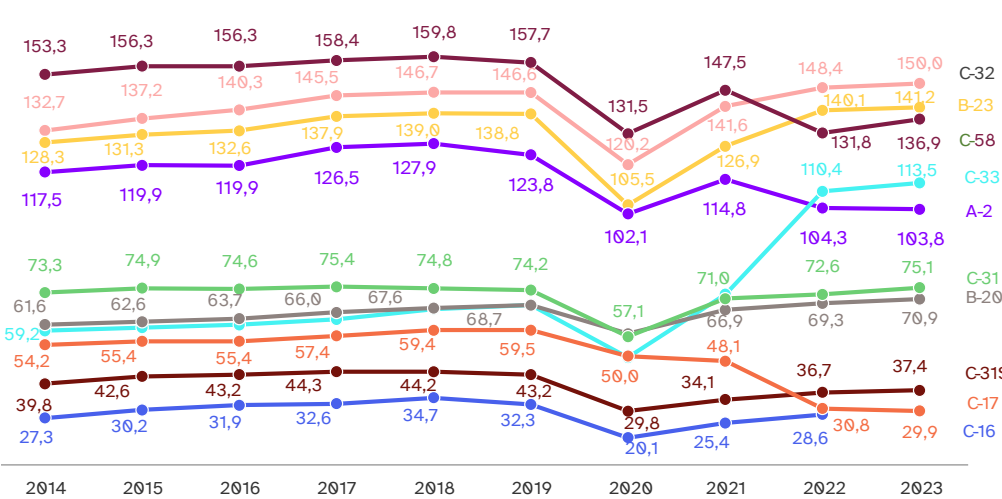
Intensitat mitjana diària (dll. - dj.) a les vies d'alta capacitat de l'àrea metropolitana de Barcelona (milers). 2014-2023
